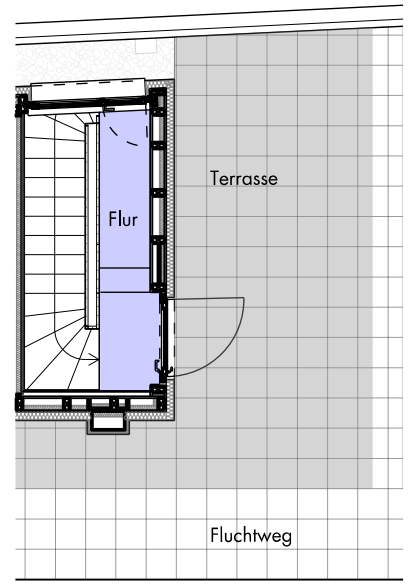
5. Obergeschoss
