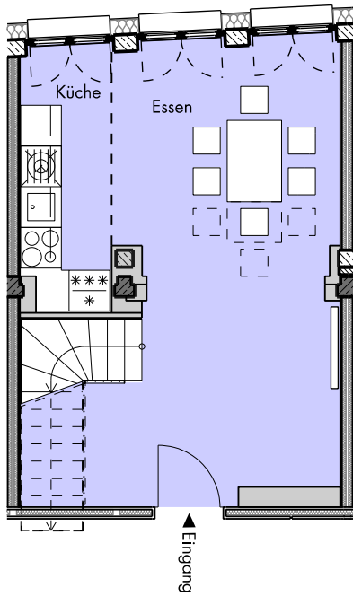
3. Obergeschoss
